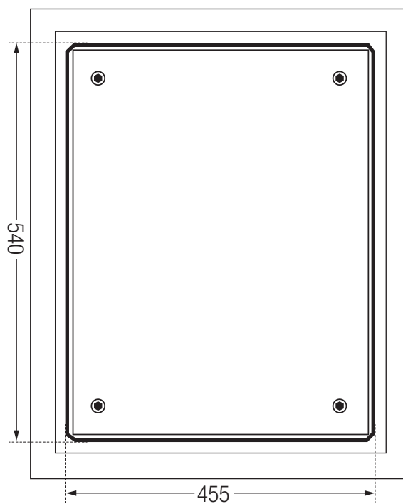
PLACA DE MONTAJE 500X600X80mm
