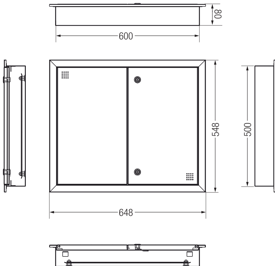
PLACA DE MONTAJE 500X600X80mm
