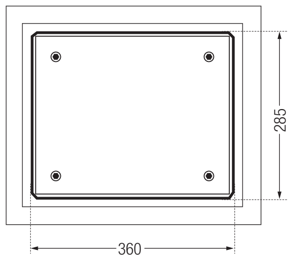
PLACA DE MONTAJE 300X400X80mm
